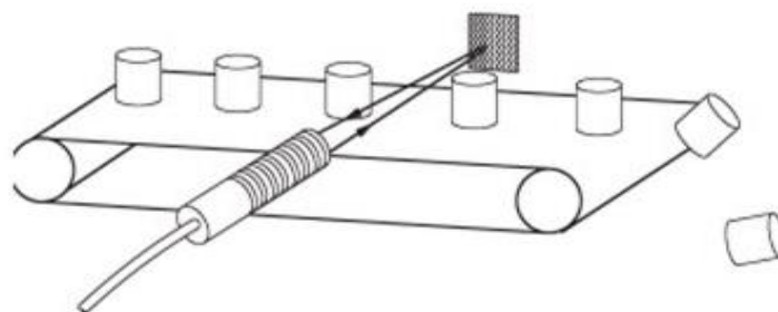
Retro-Reflective Sensors
