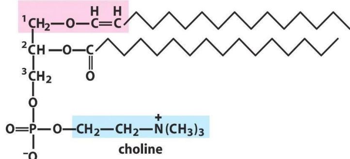
Plasmalogen
