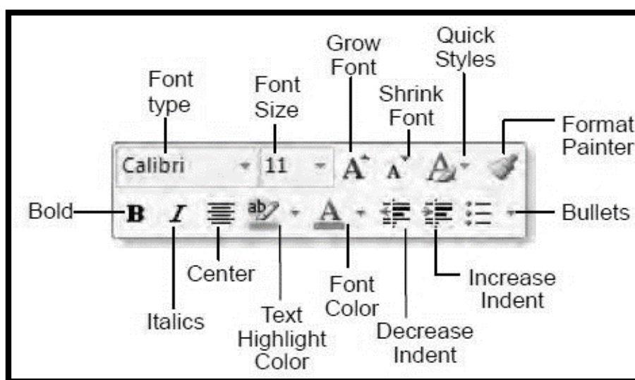
Figure 138: Mini Toolbar
