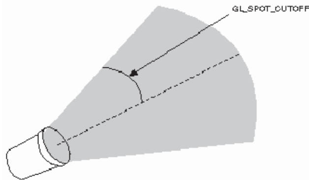
Figure 2 : GL_SPOT_CUTOFF Parameter
